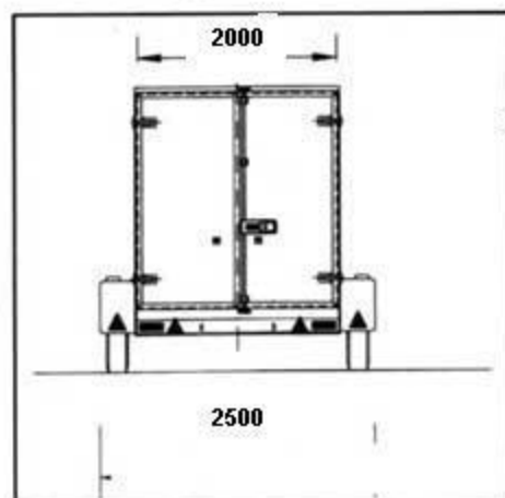
Heckansicht
